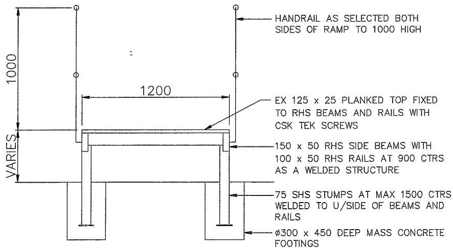
TYP RAMP SECTION 1 : 20
